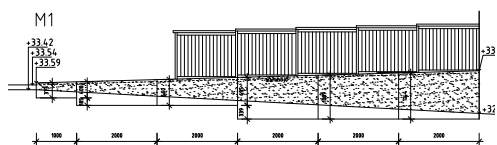
L-STÖDMURAR Skala 1:50
